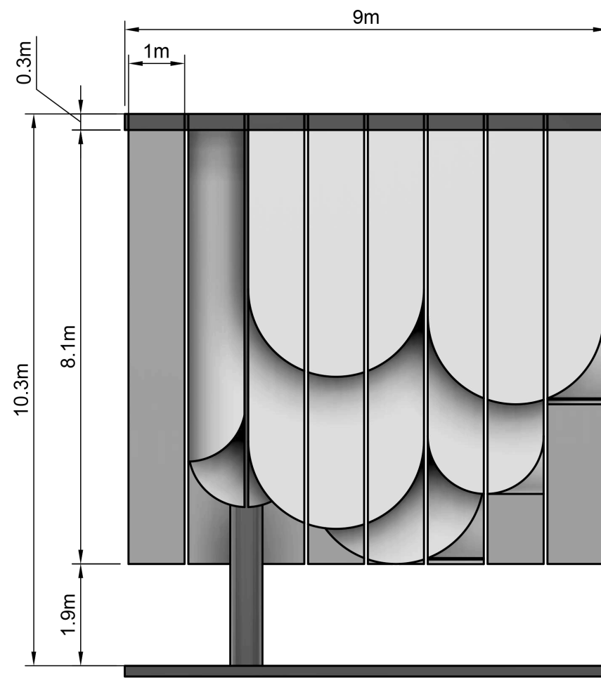
Ansicht Vorne M= 1:100
