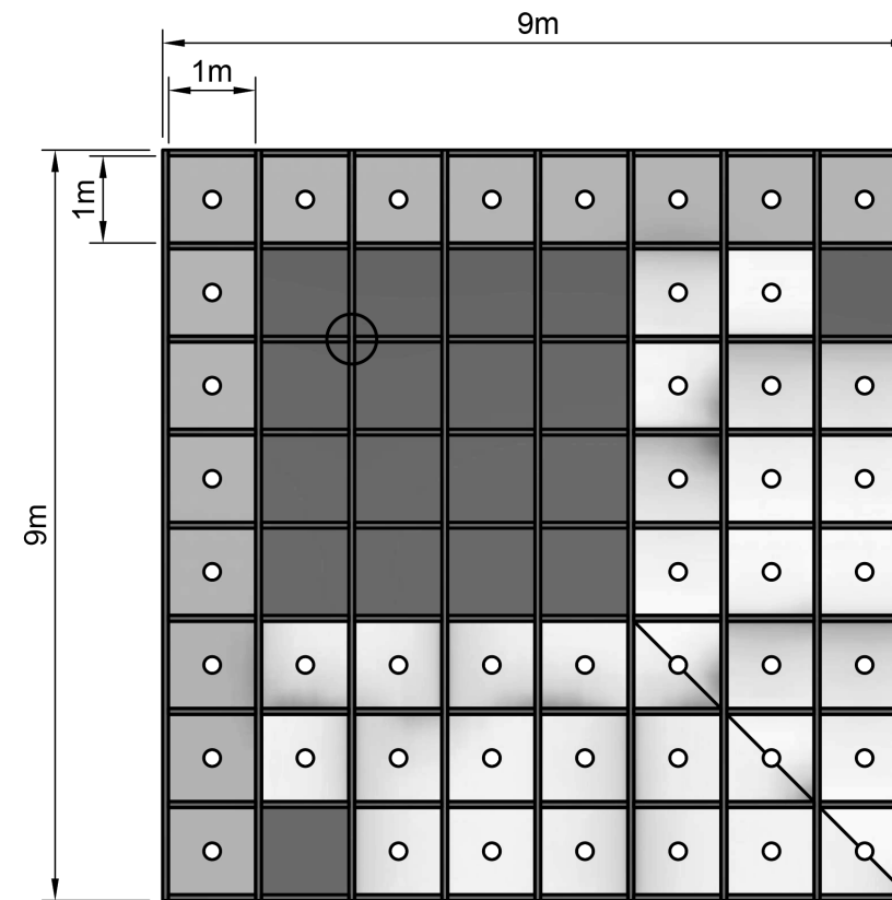
Grundriss M= 1:100
