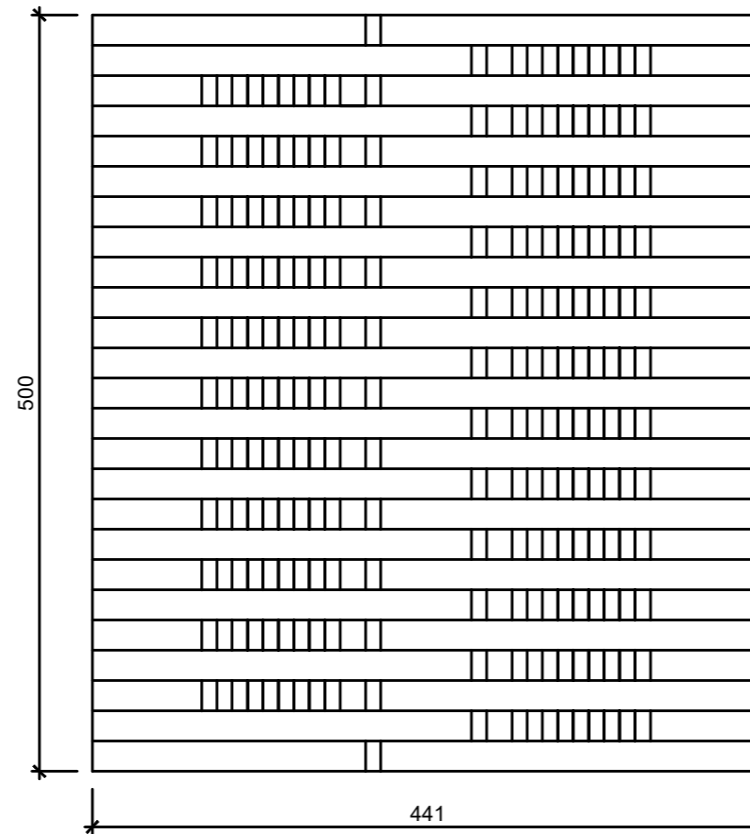
GRUNDRIS
